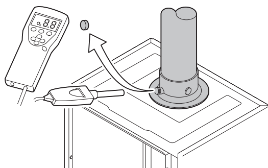
ábra26 Füstgázmérő csomak
