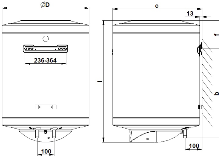
14-1. ábra Készülék méretei, felfogatási pontok
